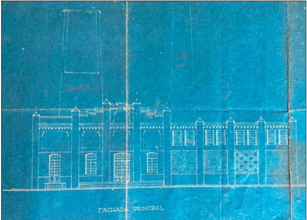
Foto: Plano Proyecto Central Eléctrica. Fachada Principal. Autor Ingeniería y Construcciones Barcelona. Fecha: 14-3-1921. Escala 1:100. Este edificio y una torre de base trapezoidal aún se conservan y deberían ser objeto de protección como patrimonio histórico local. Fuente: Archivo Empresa Medina Garvey.
